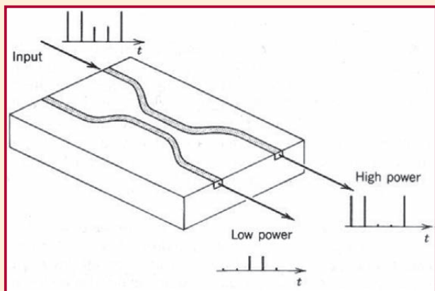
FIGURA 2. Conmutador óptica no lineal en guía de onda para técnica de multiplexado óptico por división en el tiempo.
